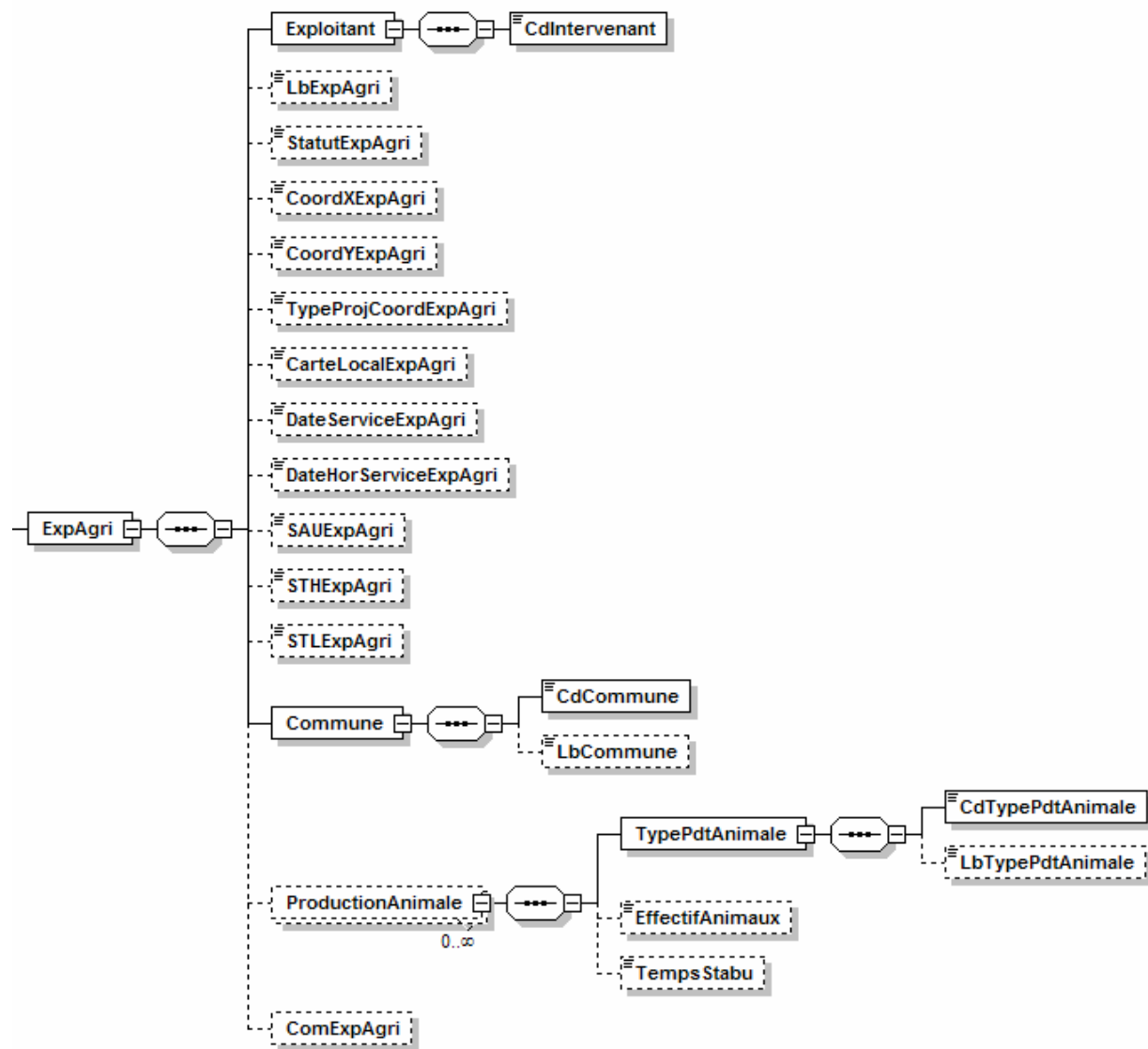
Figure 8. Diagramme représentatif de l'élément «ExAgri» (Exploitation agricole en tant qu'unité de production)
