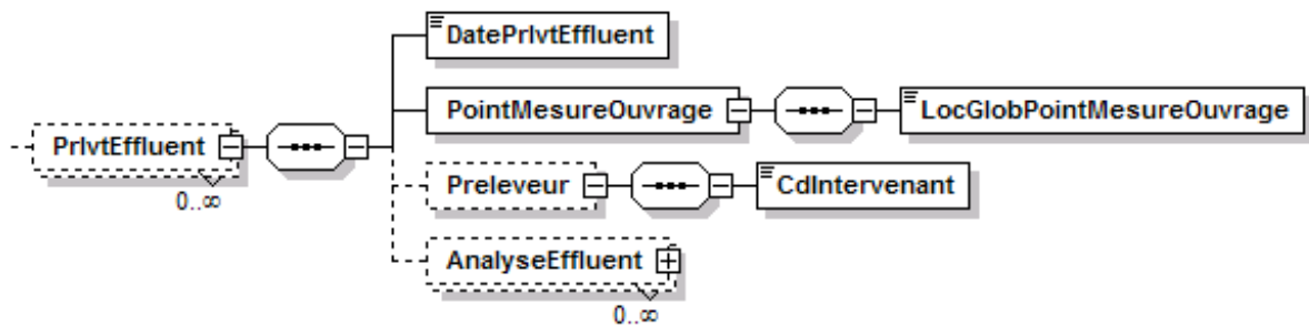
Figure 11. Diagramme représentatif de l'élément «PrlvtEffluent»
