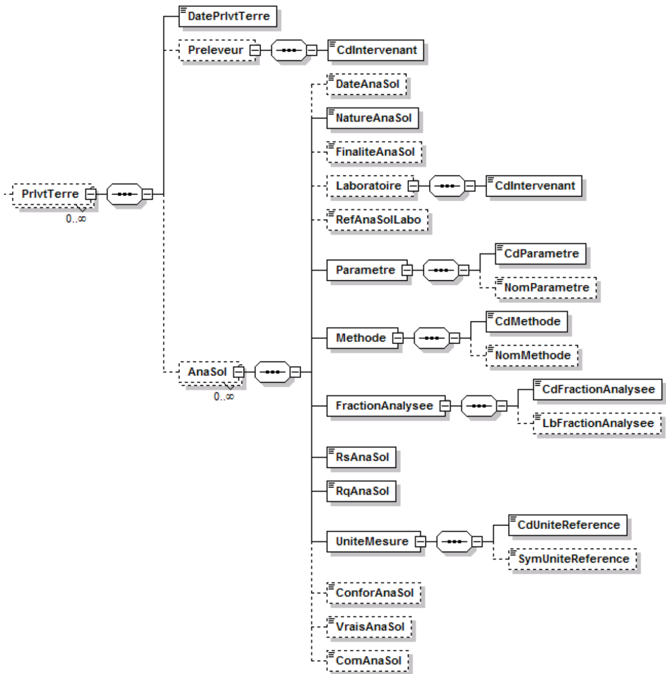
Figure 17. Diagramme représentatif de l'élément «PrvtTerre»
