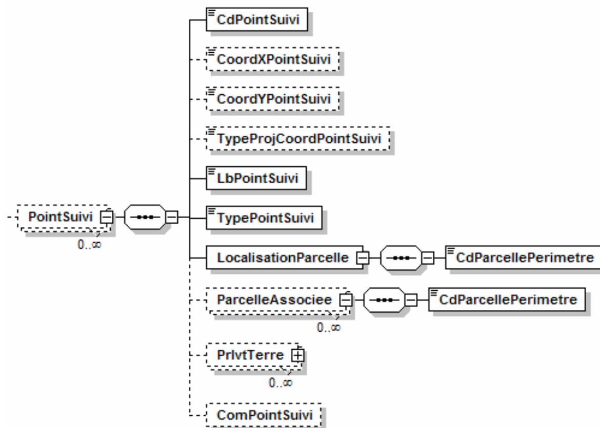
Figure 16. Diagramme représentatif de l'élément «PointSuivi»
