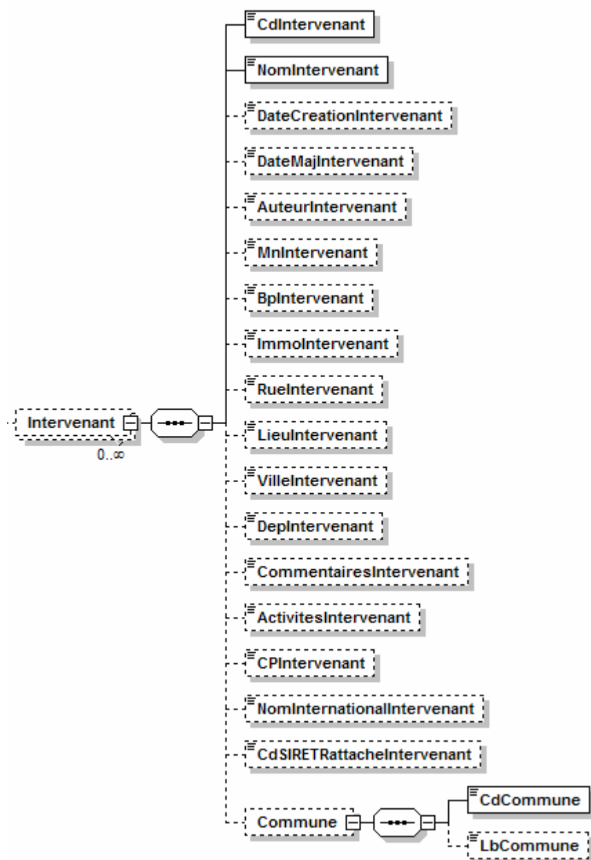
Figure 3. Diagramme représentatif de l'élément XML <Intervenant>
