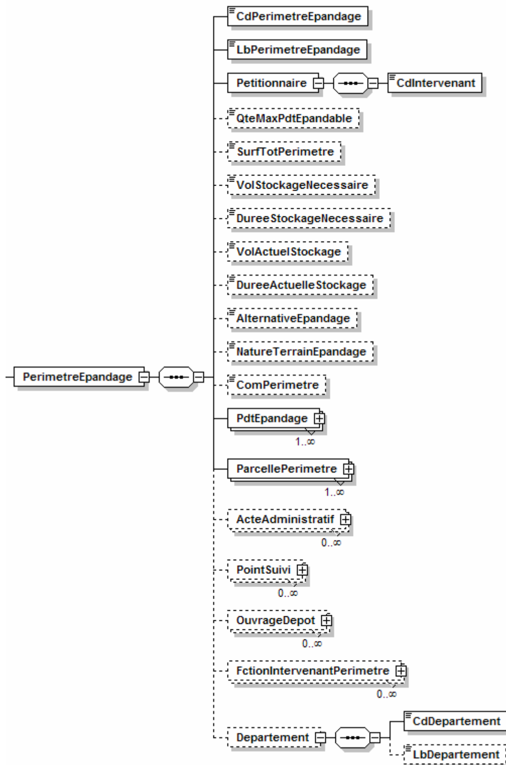
Figure 9. Diagramme représentatif de l'élément <PerimetreEpannage>
