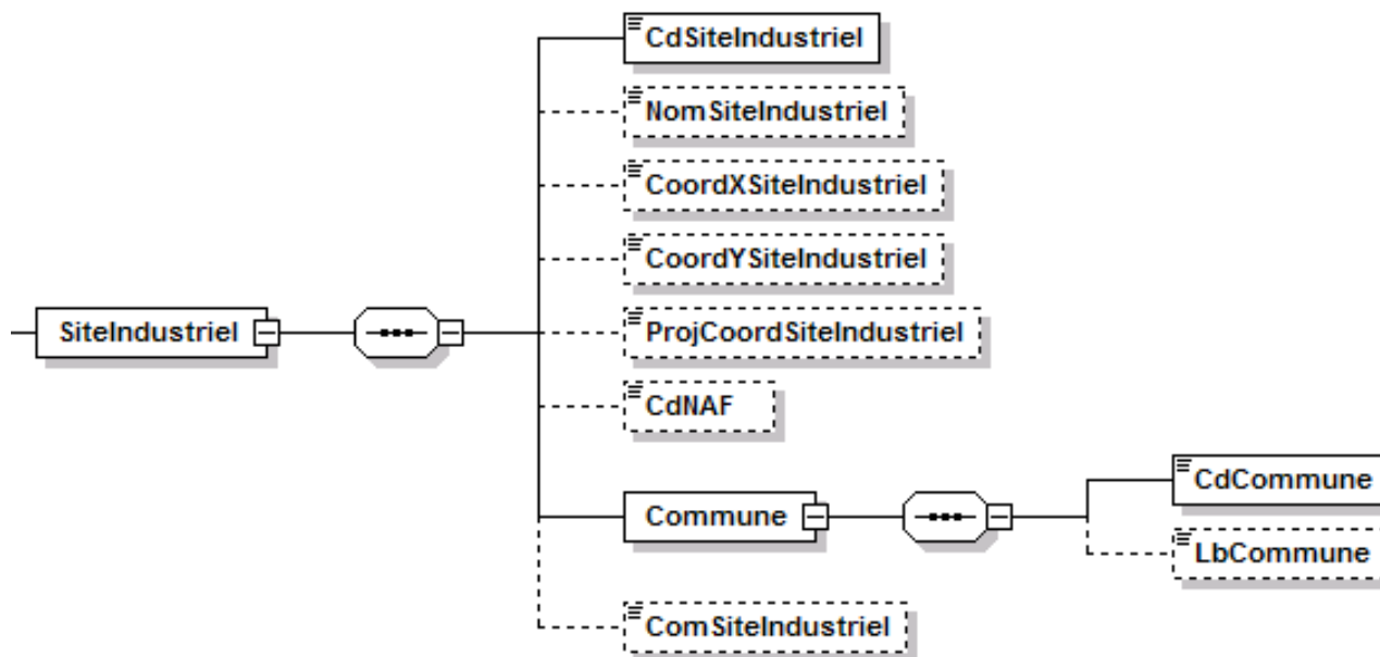
Figure 7. Diagramme représentatif de l'élément «SiteIndustriel»
