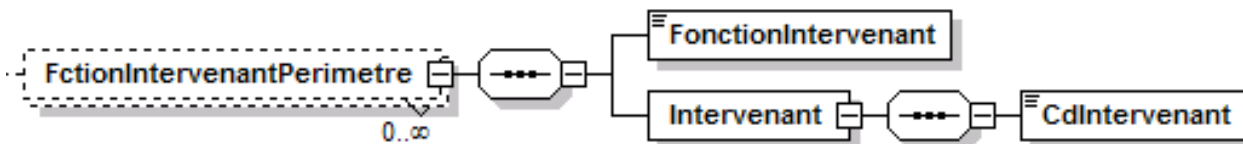
Figure 20. Diagramme représentatif de l'élément «FctionIntervenantPerimetre»
