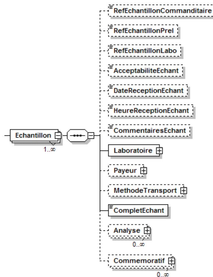
Figure 11. Diagramme représentatif de l'élément XML <Echantillon>
