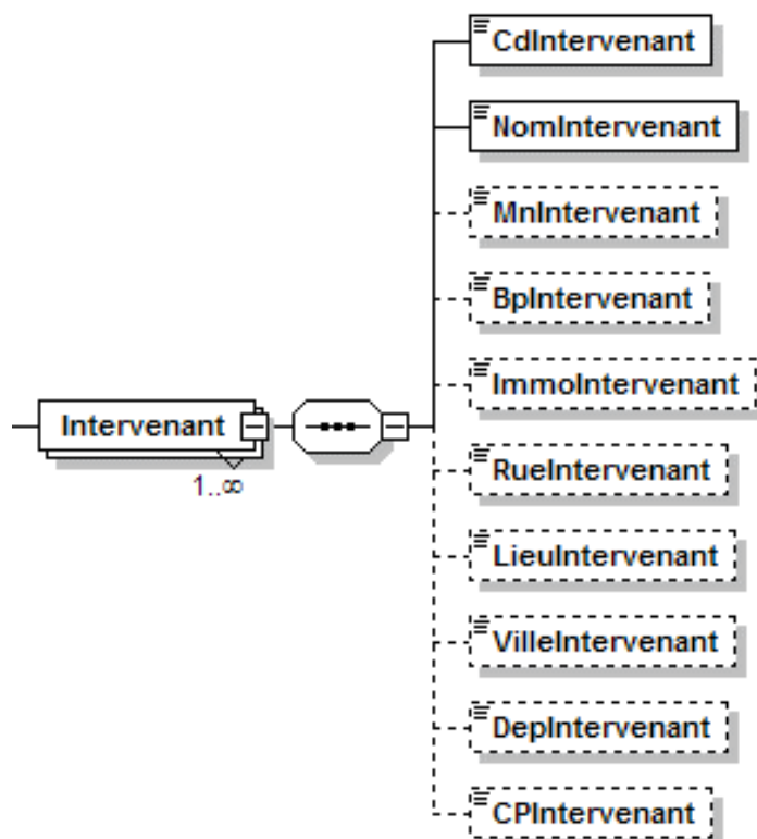
Figure 5. Diagramme représentatif de l'élément XML <Intervenant>
