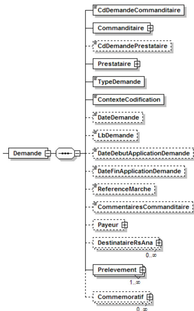
Figure 8. Diagramme représentatif de l'élément XML <Demande> (contexte d'échange « 1 »)
