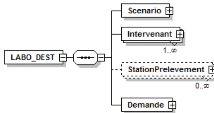
Figure 1. Diagramme représentatif de l'élément racine <LABO_DEST>
