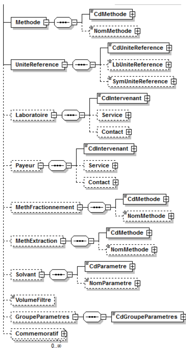
Figure 12. Diagramme représentatif de l'élément XML <Analyse>
