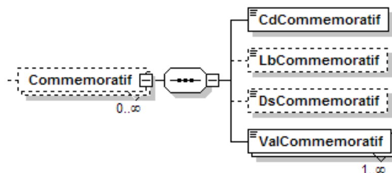
Figure 14. Diagramme représentatif de l'élément XML <Commémoratif>
