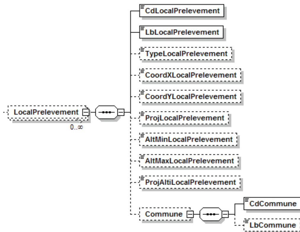
Figure 7. Diagramme représentatif de l'élément XML <LocalPrelevement>
