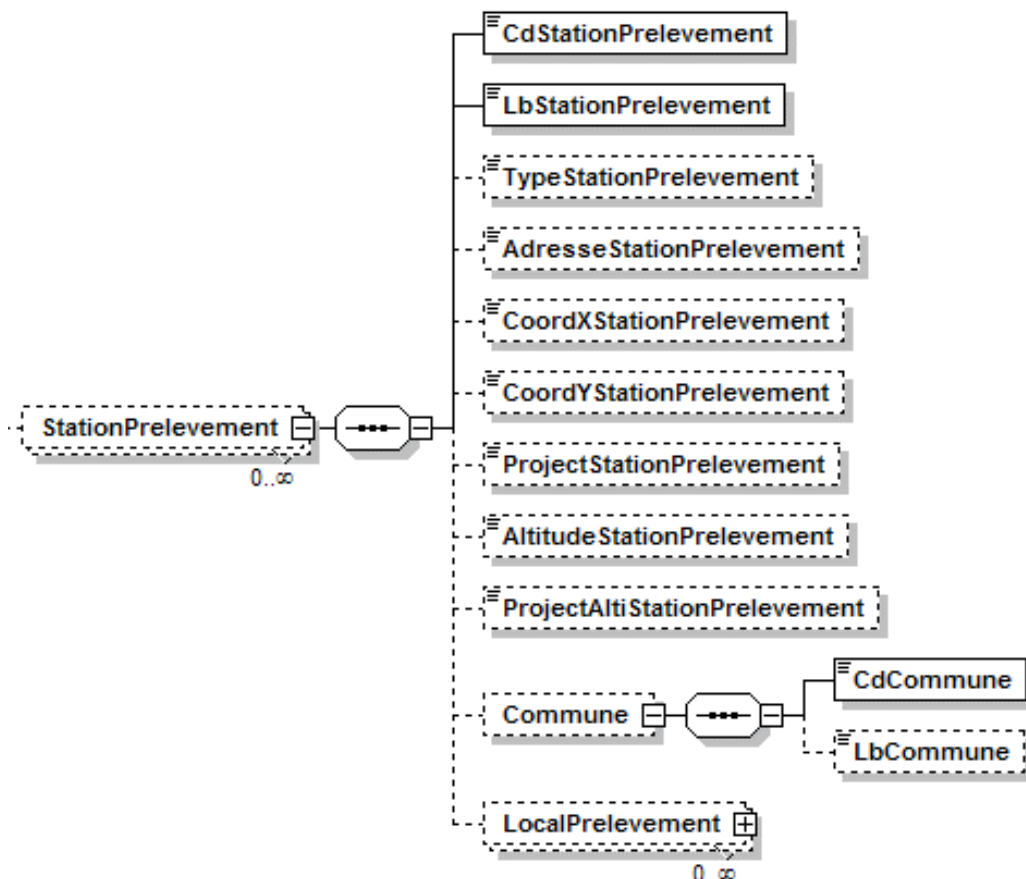
Figure 6. Diagramme représentatif de l'élément XML <StationPrelevement>
